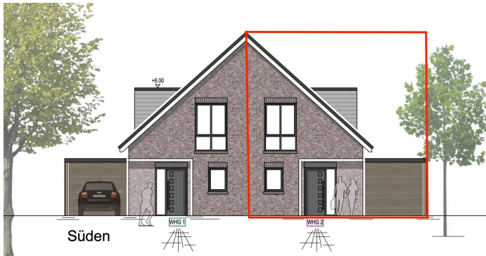
Ansicht WHG 2
